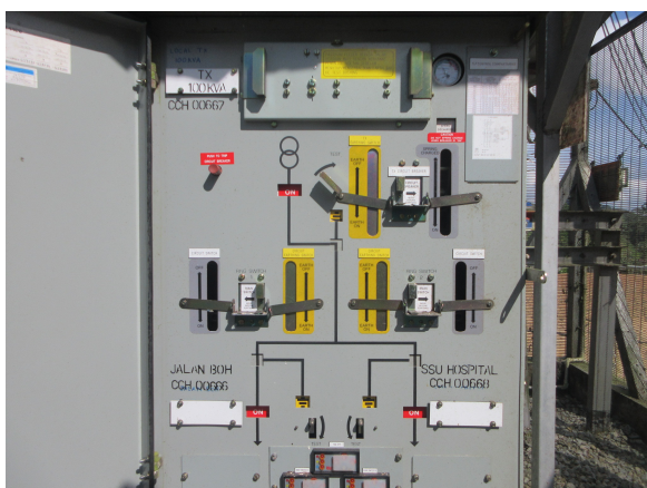
SWITCHGEAR
